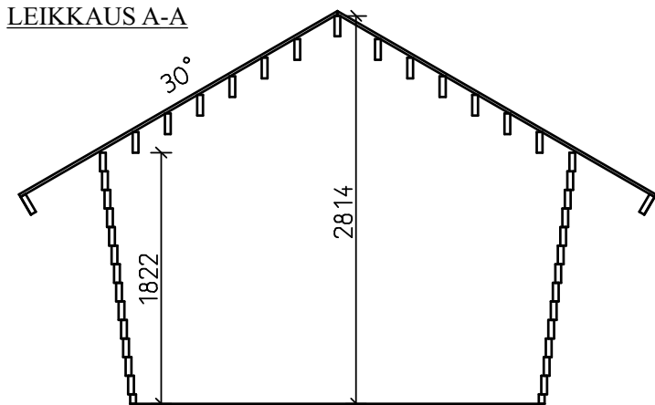
LEIKKAUS A-A
