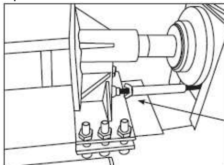
KUVA 8 Säädä haluttu halkaisupituus siipimutterilla pöllipituuden mukaiseksi.
