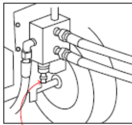
Maksimipaineen rajoitinruuvi
