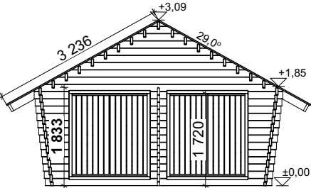
LEIKKAUS 1:100
