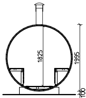
LEIKKAUS
