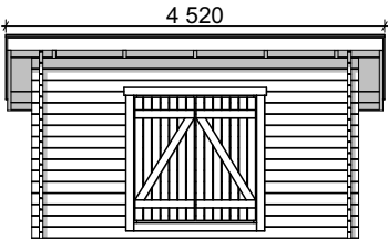
Fasad 1:100
