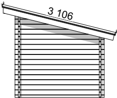
Fasad 1:100
