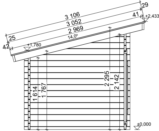
Snitt 1:50
