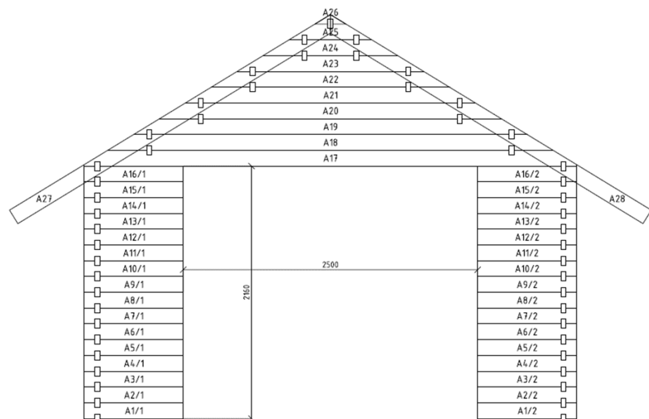
Стена А
