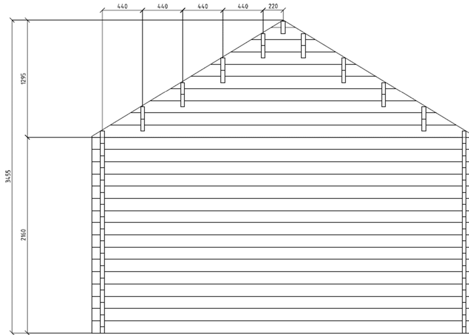
Разрез 1-1
