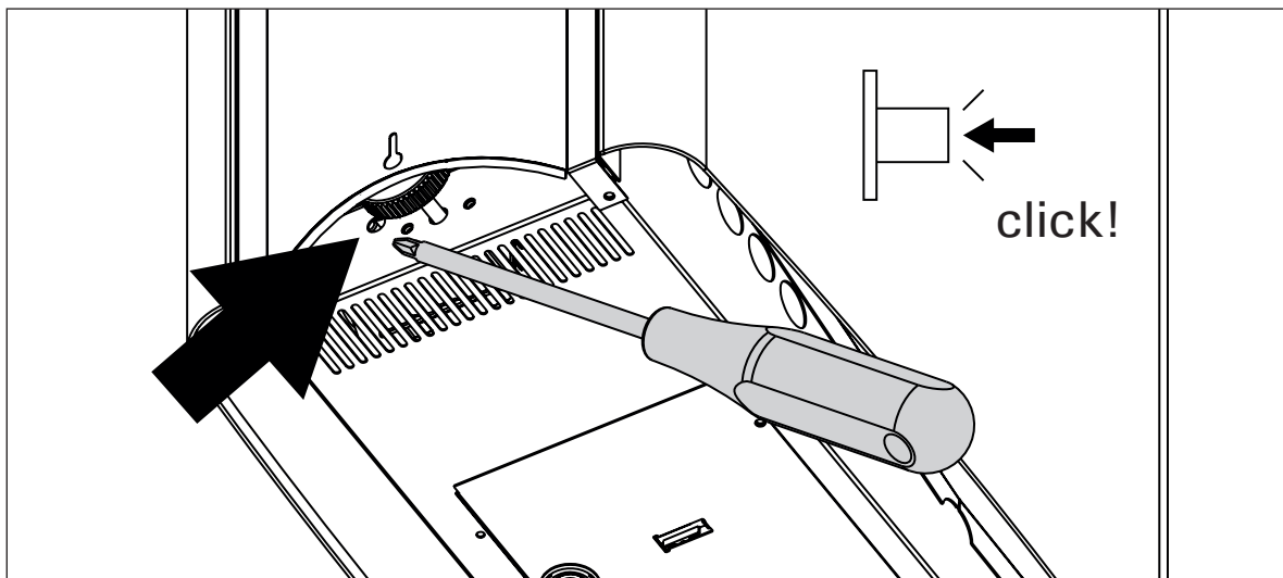
Figure 12. Réinitialisation de la sécurité-surchauffe
