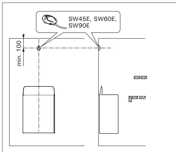
Рисунок 6. Установка датчиков (все размеры приведены в миллиметрах) Joonis 6. Anduri paigaldamine (kõik mõõtmised millimeetrites)
