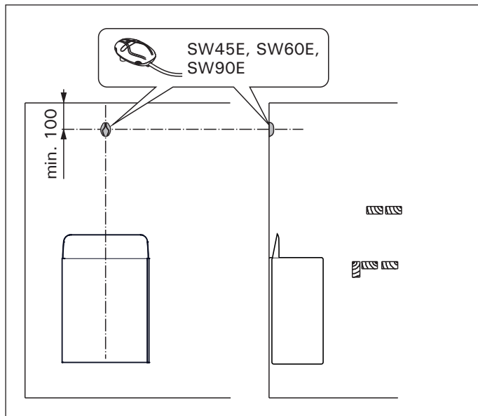
Kuva 6. Anturin asentaminen (mitat millimetreinä) Bild 6. Montering av givaren (mått i millimeter)
