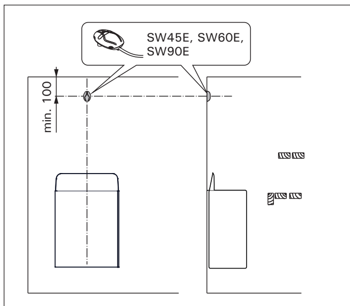
Figure 6. Installation du capteur (toutes les dimensions sont fournies en millimètres) Rys. 6. Instalowanie czujników (wymiarów w milimetrach)
