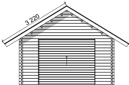
Julkisivu _____
