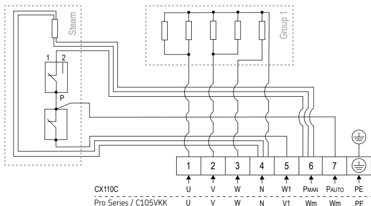
Bild 5. Kopplingsschema QU100S
