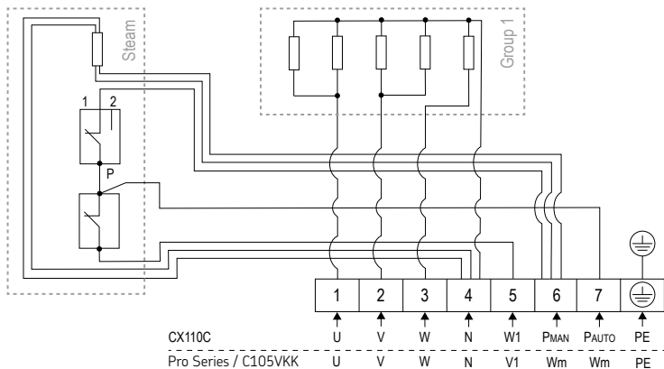
Kuva 5. Kytentäkaavio QU100S
