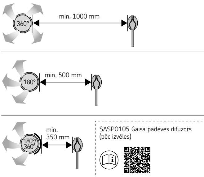
9. attēls. Minimālais attālums no gaisa padeves lūkas līdz temperatūras sensoram
