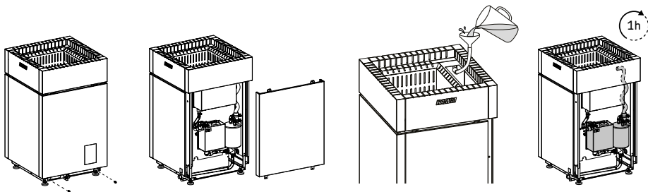
Kuva 12. Kalkinpoisto sitruunahappoliuoksella
