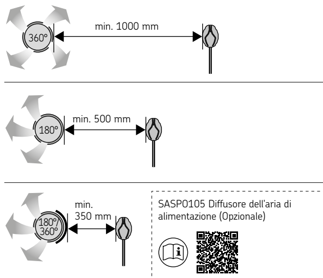
Figura 9. Distanza minima tra lo sfianto dell'aria di alimentazione e il sensore di temperatura.
