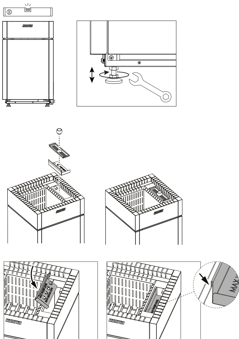
Рисунок 2. Установка каменки
