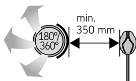
Kuva 9. Tuloilmaventtiilin vähimmäisetäisyys lämpötila-anturiin
