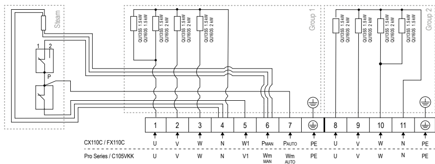
Obrázek 6 Schéma zapojení QU135S, QU160S
