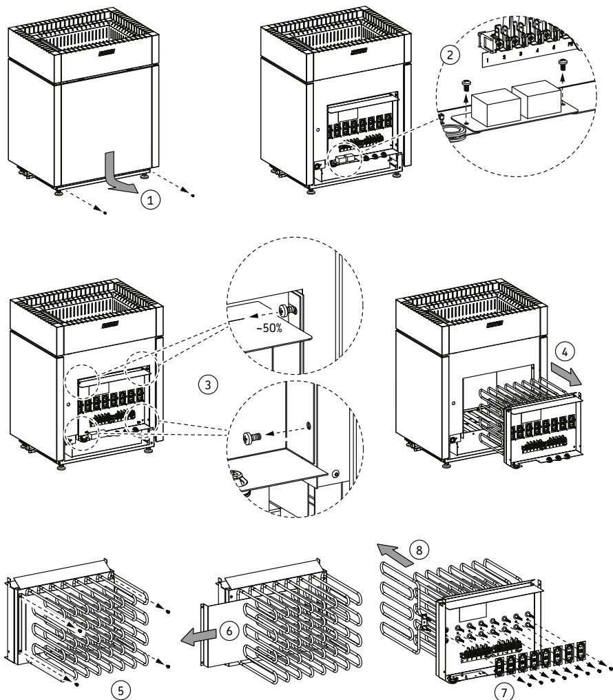
Bild 13. Byta värmeelement
