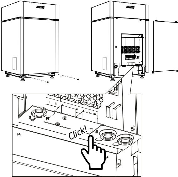
Kuva 14. Höyrystimen ylikuumenemissuojan kuittaus
