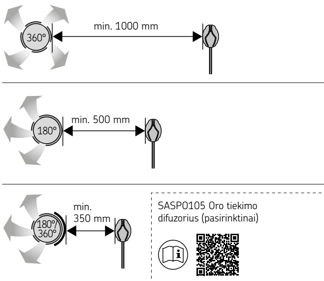
9 pav. Mažiausias atstumas nuo tiekiamo oro ventiliacijos angos iki temperatūros jutiklio
