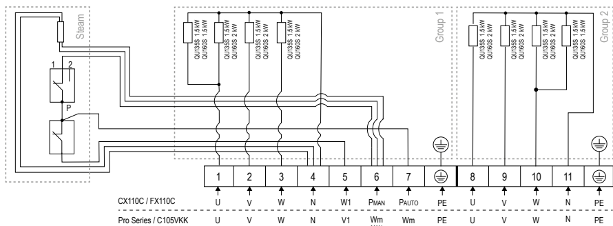
Slika 6. Shema ožičenja QU1355, QU1605
