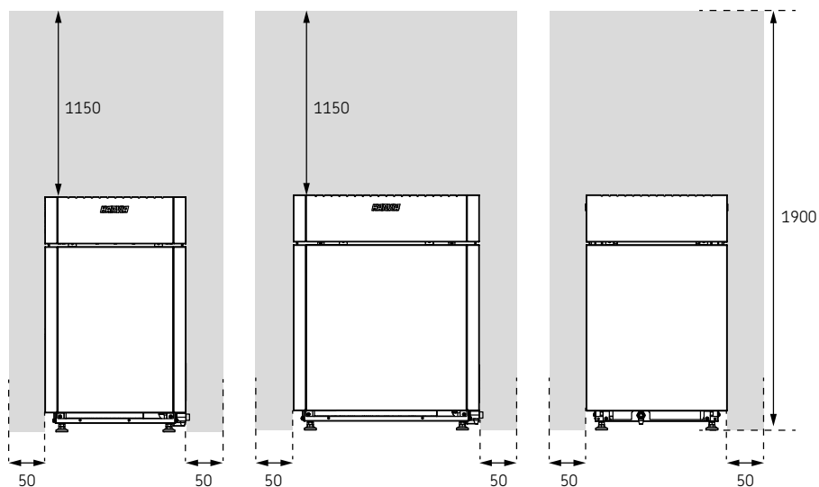
Рисунок 1. Безопасное расстояние
