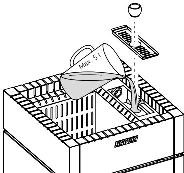
Kuva 10. Vesisäiliön täyttö
