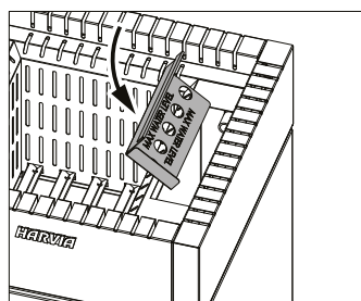
Figuur 2. Installatie saunakachel
