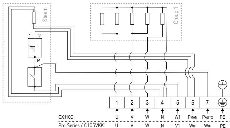
Slika 5. Shema ožičenja QU1005
