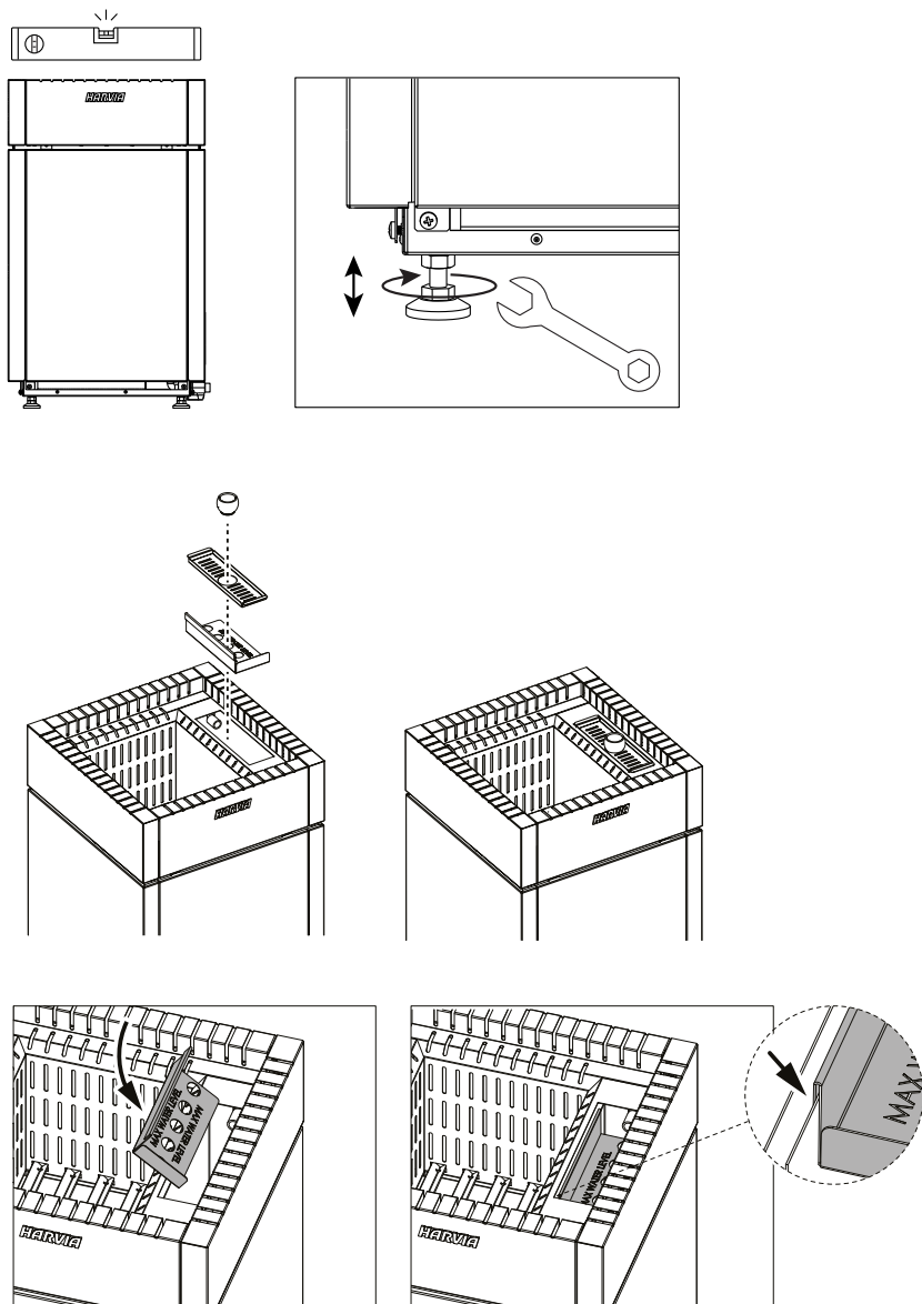
Joonis 2. Kerise paigaldamine
