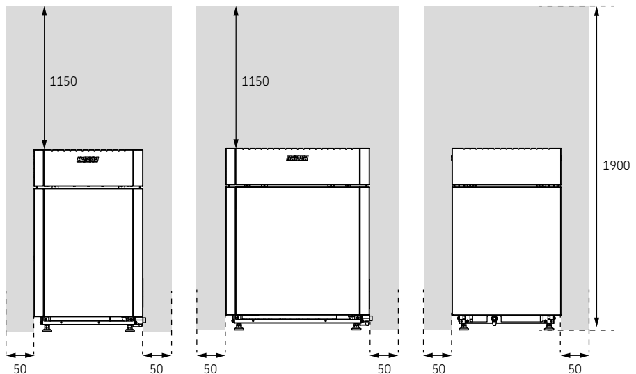
Abbildung 1. Sicherheitsabstände
