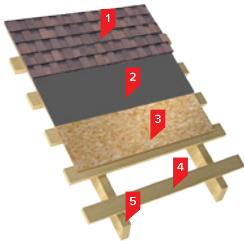
Eristämätön kattorakenne
