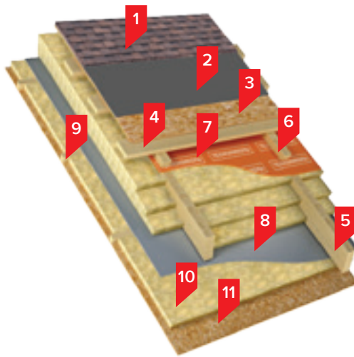
Eristetty kattorakenne
