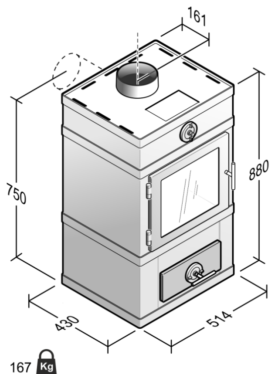
Grundmodel Varenummer 1100
